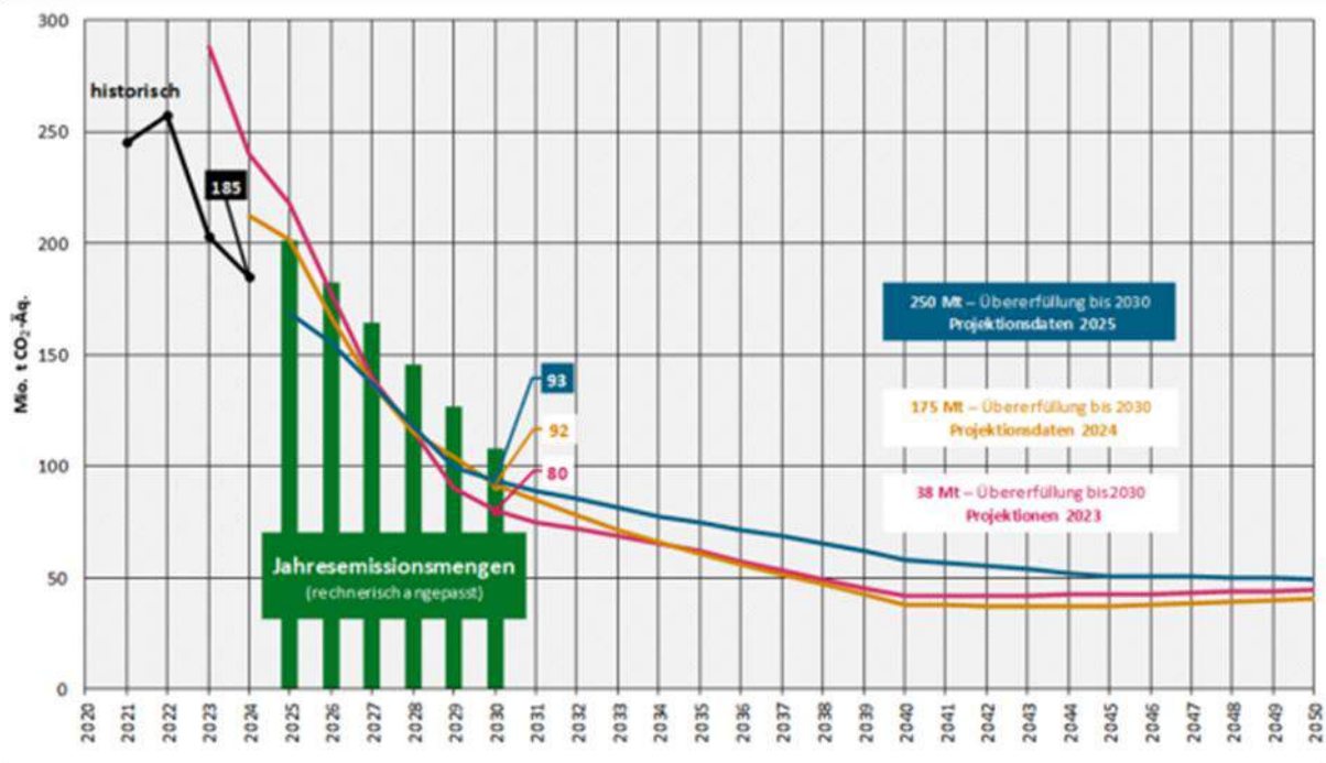
Abbildung 6: Entwicklung der Treibhausgasemissionen im Sektor Energiewirtschaft
