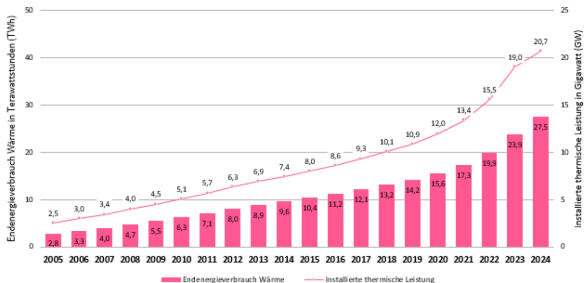
Abbildung 21: Entwicklung des Endenergieverbrauchs von oberflächennaher Geothermie und Umweltwärme
